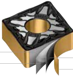
Abb.: Schichtaufbau TTG
